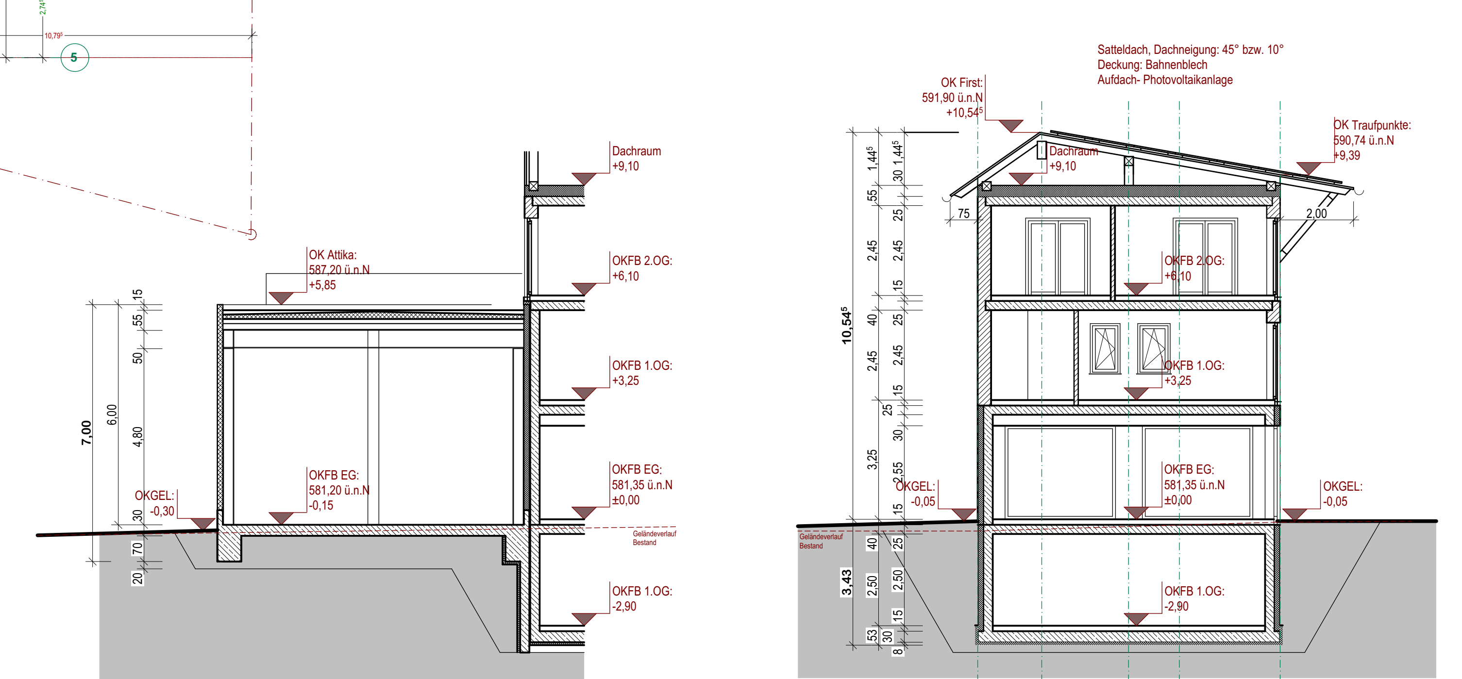
Schnitt Busgarage
