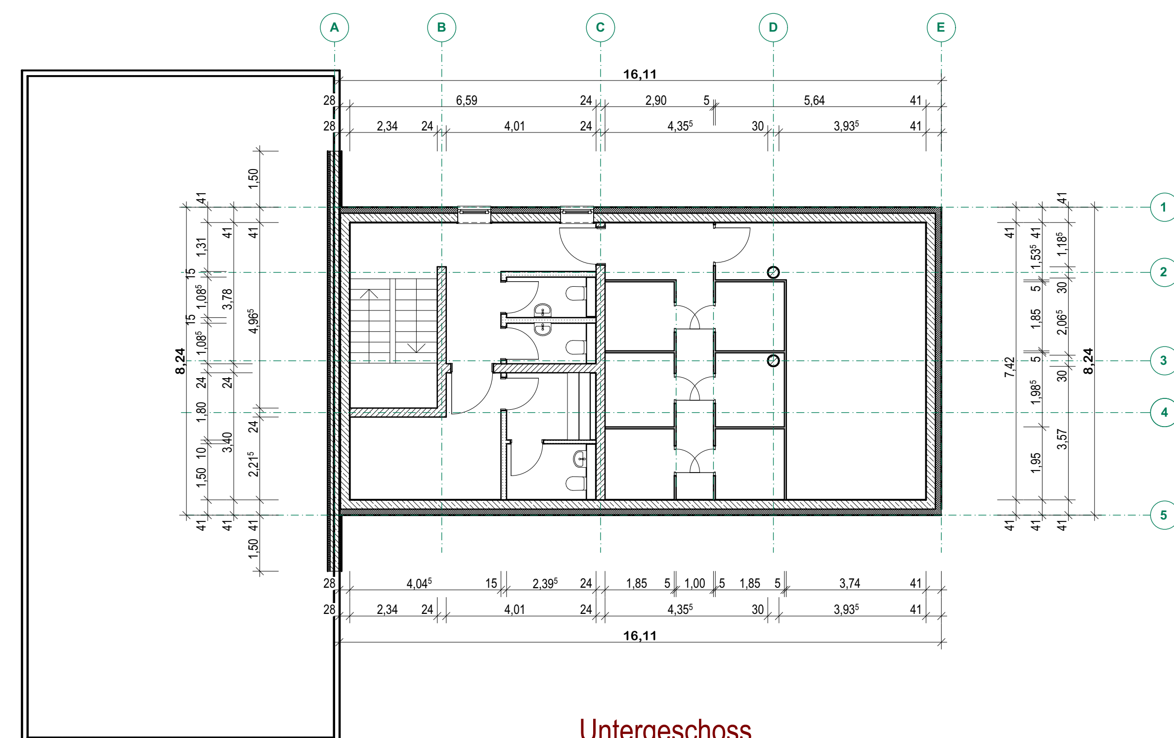
Untergeschoss
